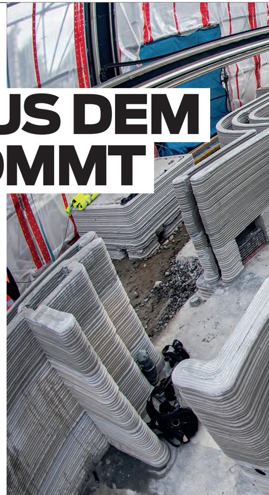
vorn mit dabei: Das erste deutsche Wohnhaus aus dem 3-D-Drucker entsteht hier.
